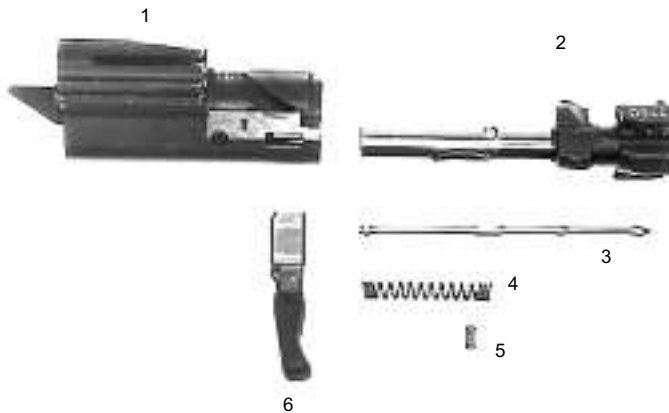
Bild 4: Verschluss zerlegt
