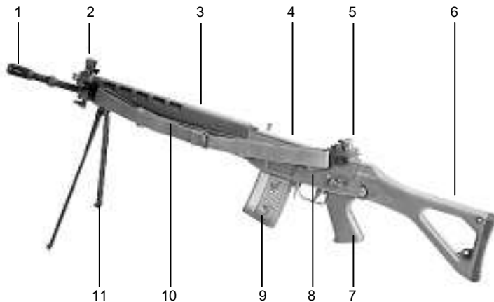
Bild 1: Hauptbestandteile des 5,6 mm Stgw 90
