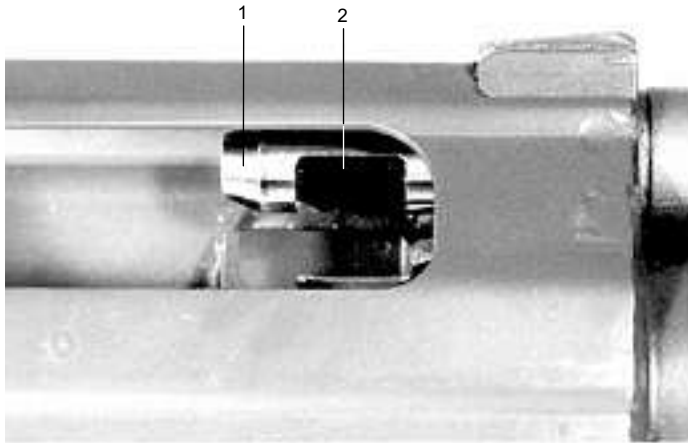
Bild 15: Gasstange einbauen: richtige Lage der Arretiernute
