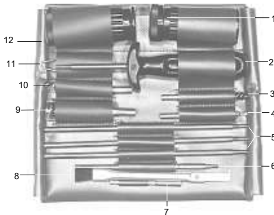
Bild 13: Putzzeug
