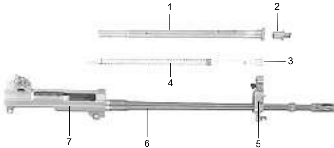
Bild 5: Gaseinheit mit Lauf und Verschlussgehäuse
